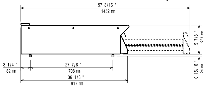
Boven aanzicht
